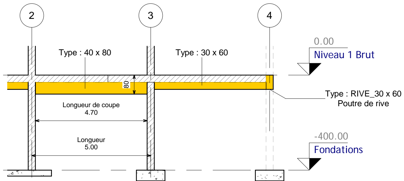
COUPE SUR POUTRES
